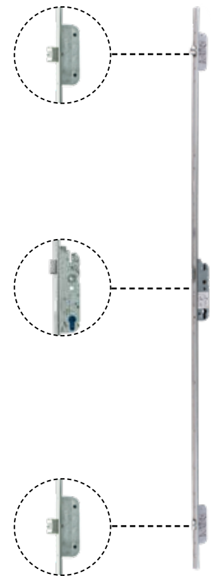
GU automatikus zár (autómata retesz ajtók esetén az elektromos zárfogadó nem kom- patibilis!)
